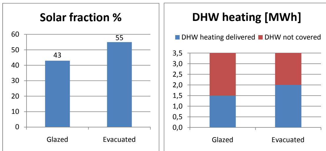
Figura 5.4.1. Comparación de la fracción solar y ACS suministrada para los diferentes tipos de colectores para el caso finés.
