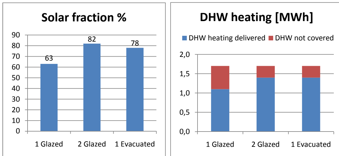
Figure 5.4.2. Comparación de la fracción solar y ACS suministrada para las diferentes soluciones para el caso de Madrid.
