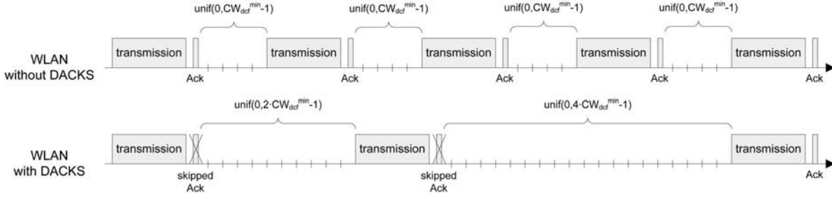
Fig. 1. DACKS technique.
