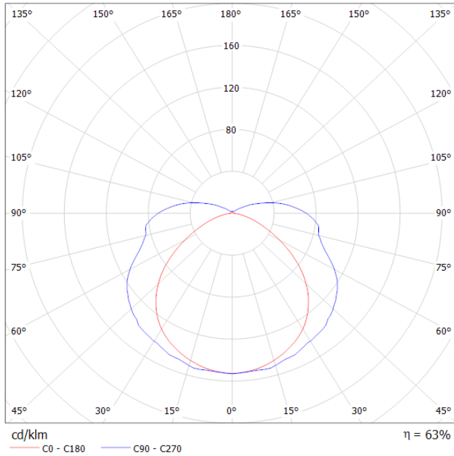
INDAL Z7102202sM2 400139EL / Diagrama de densidad lumínica
