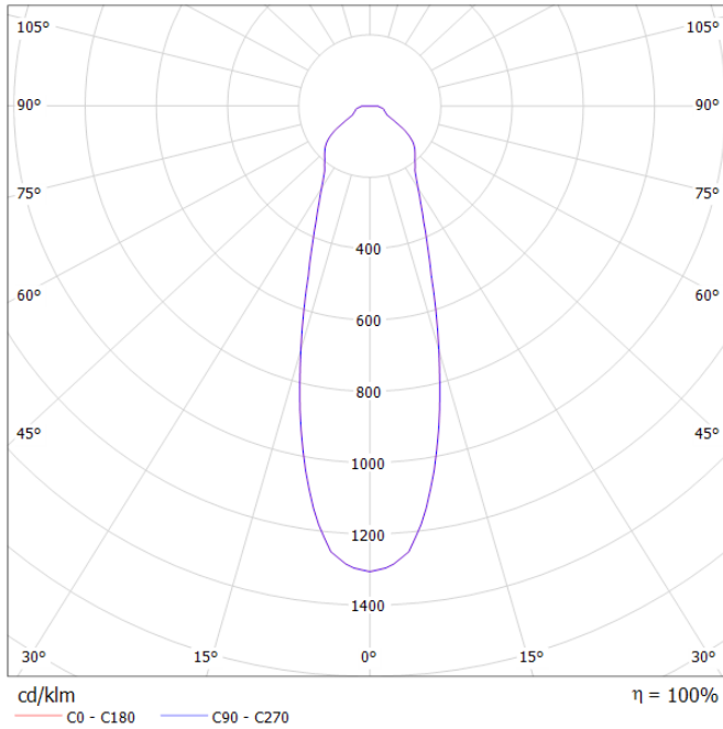
INDAL Z2052901 3300 / Diagrama de densidad lumínica
